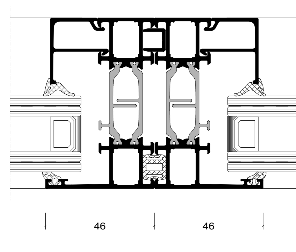
Verborgen koppeling
