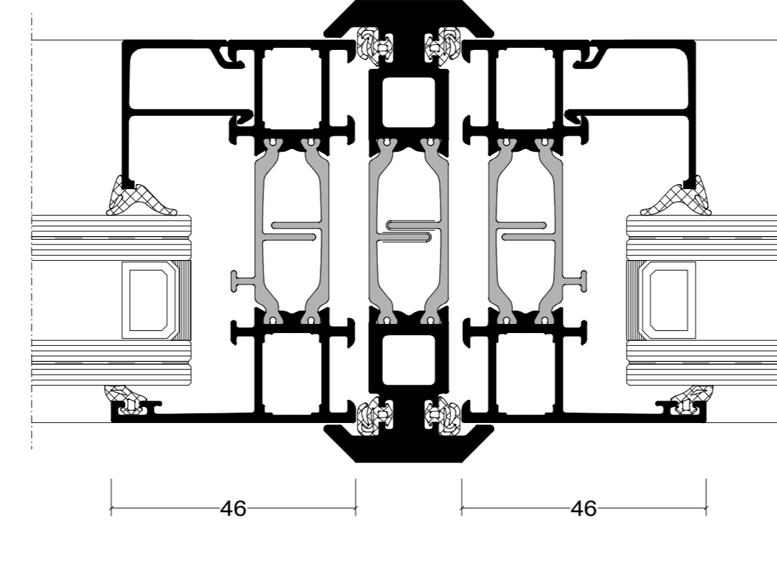
Vlakke koppeling
