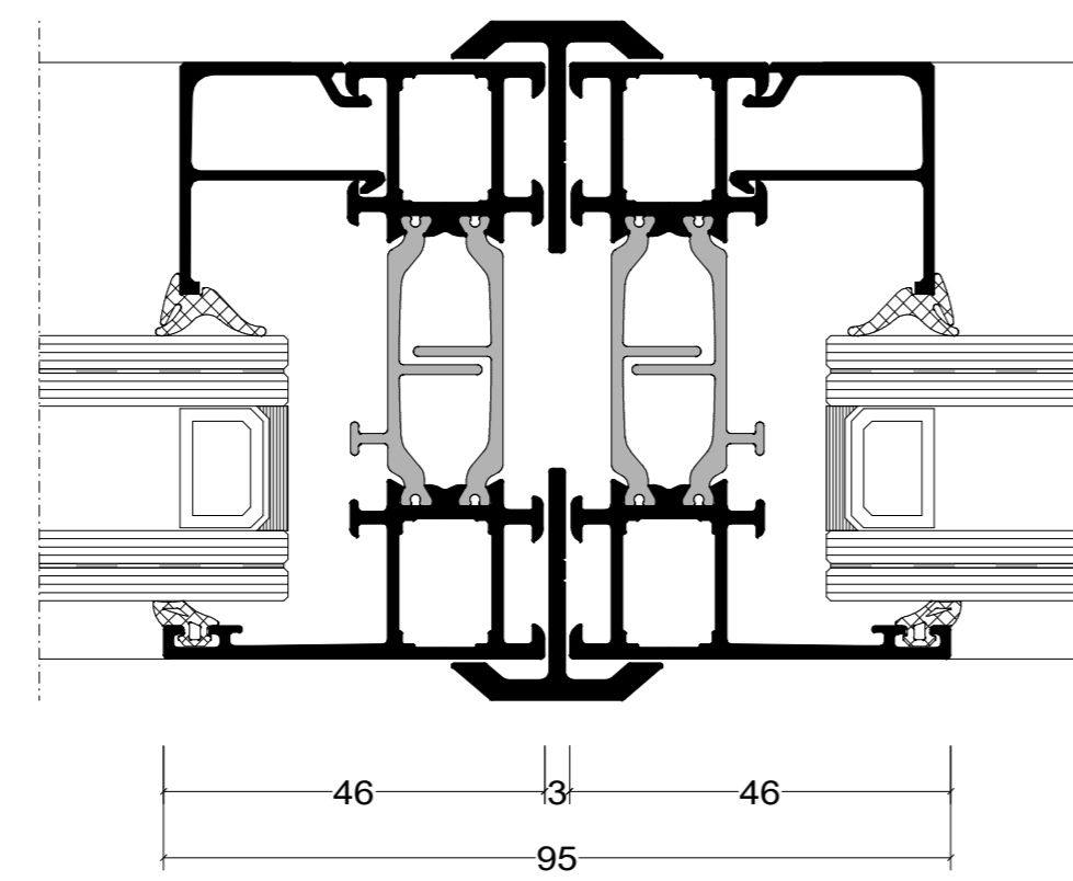
Losse koppeling
