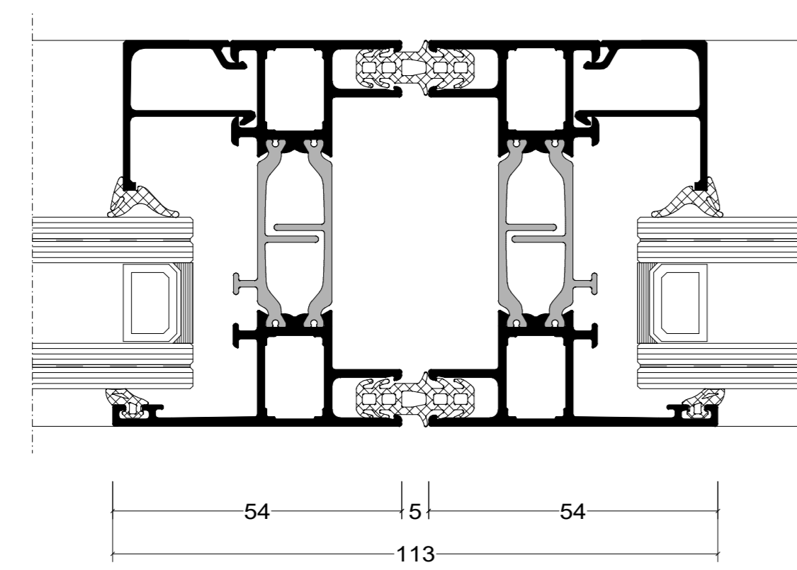
Dilatatie koppeling
