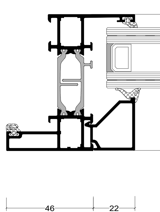
Buitenbeglazing raam
