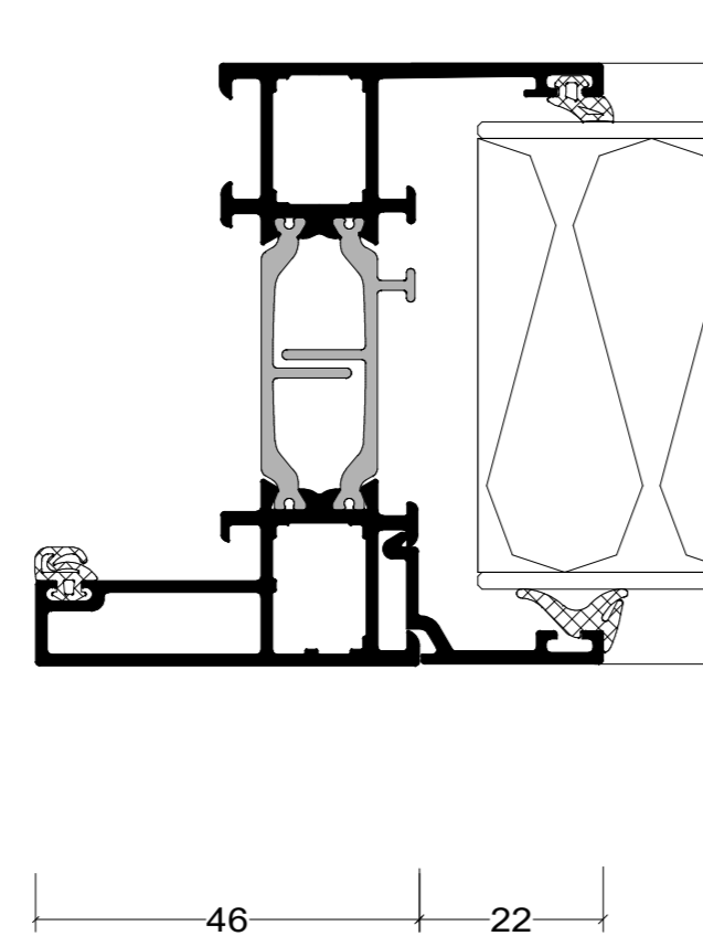
Buitenbeglazing raam
